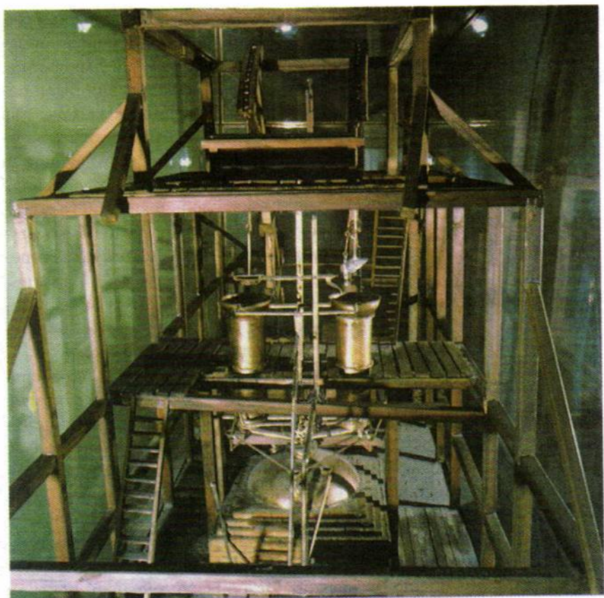
Макет паровой машины И. Ползунова.
